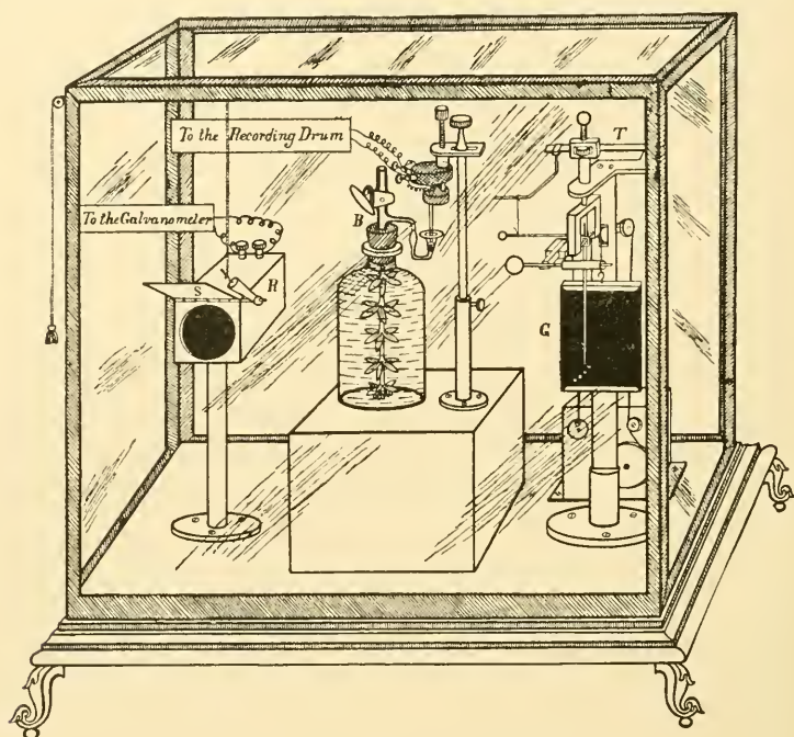
FIG. 43. The Complete Apparatus
