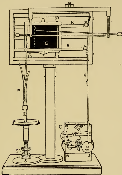
FIG. 3. Complete apparatus.
